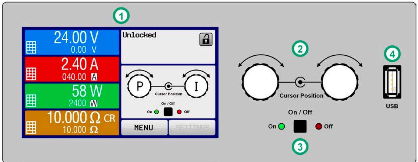
图 6- 控制面板
