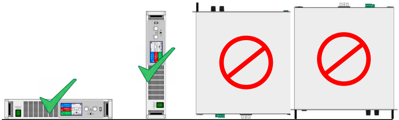
直立面
