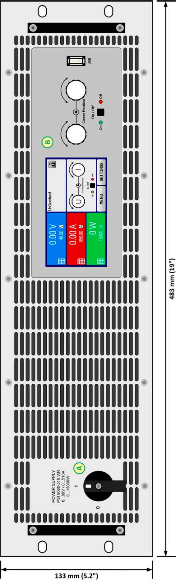
图 1 - 前视图
